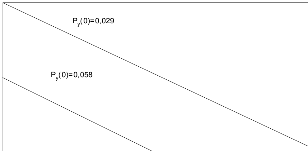
Рис. А-3. Область допустимых значений частоты пролетов воздушных судов в одном и встречных направлениях, основанная на взаимоизменении параметров с вероятностью бокового перекрытия, P_y(0) , для двух различных значений P_y(0)
